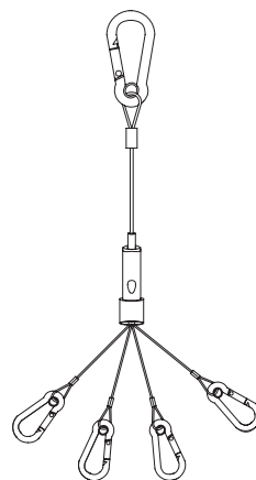
Pendant Rope
